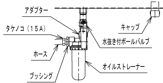
送油口詳細図
