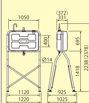
※カッコ内は250型の寸法です。
