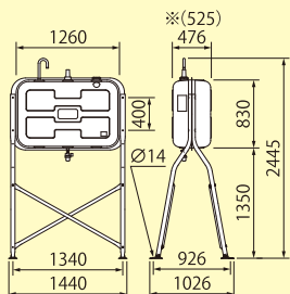
KS3-490KJ (Q) / 500KJ (Q)
