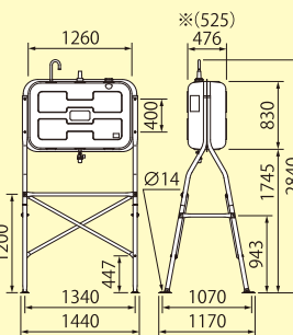
KS3-490HJ (Q) / 500HJ (Q)
